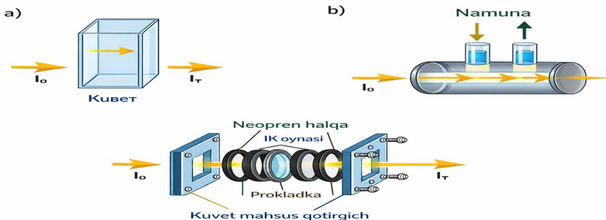
1-rasm. O'tkazish o'lchov katakchalari: (a) suyuq UV katakcha, (b) gazlar va suyuqliklar uchun oqim katakcha; (c) olinadigan suyuq IQ katakcha [2]
