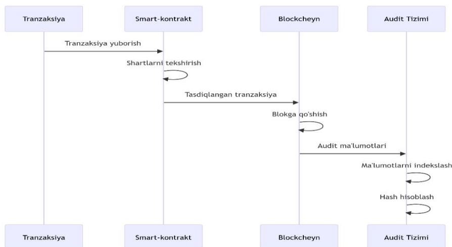
4-rasm. Blockchain asosidagi audit izi va tranzaksiya tasdiqlash jarayoni
